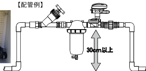
【配管例】
